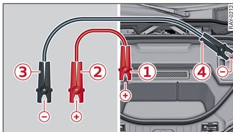
图 135 连接辅助启动电缆
