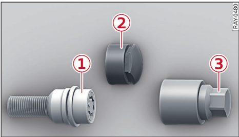
图 131 防盗型车轮螺栓及封盖和适配接头
