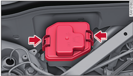
图 139 前舱右侧：保险丝盒
