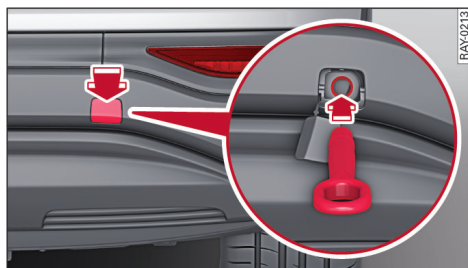
图 137 后保险杠：拧入拖车环
