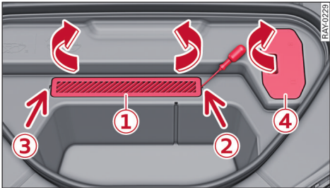
图 122 前舱：充电极点的盖子：① 正极 / ④ 接地点
