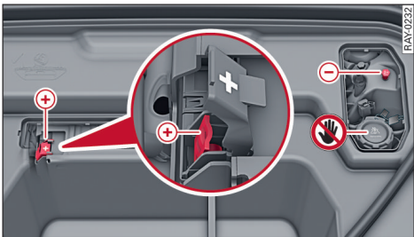
图 123 前舱：充电装置或辅助启动电缆的接口
