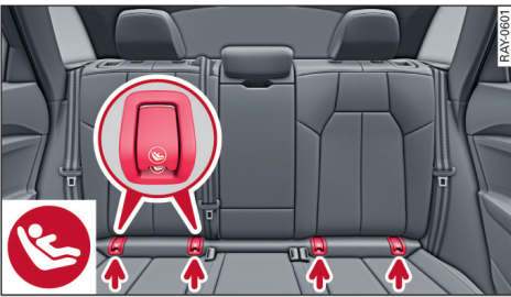
图 47 后座长椅：下部 ISOFIX 固定座
