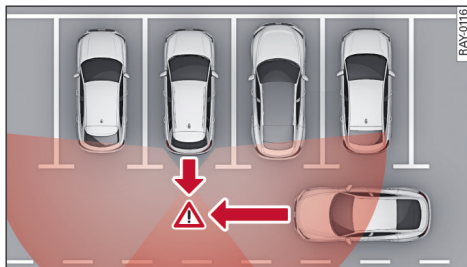
图 105 装有后方交通穿行辅助系统时的感应器探测范围
