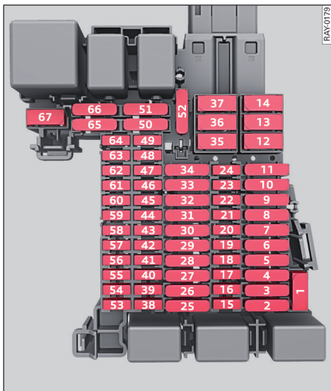
图 144 行李厢左侧：保险丝座
