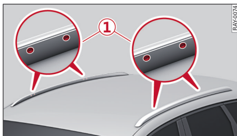
图 60 车顶行李架饰条：固定点
