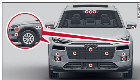
图 72 前部：感应器和摄像头
