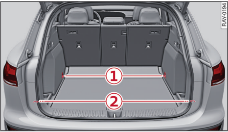
图 59 行李厢：固定环的布置
