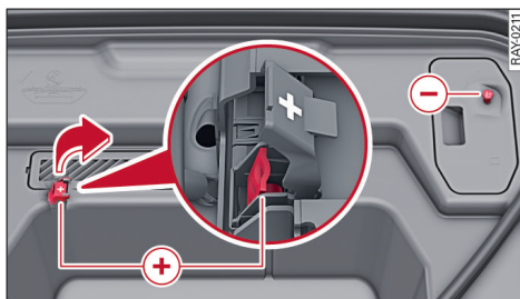
图 134 前舱：辅助启动电缆或充电装置的接口
