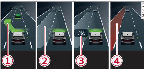
图 95 组合仪表：导航辅助驾驶系统：监督式车道变换功能显示
