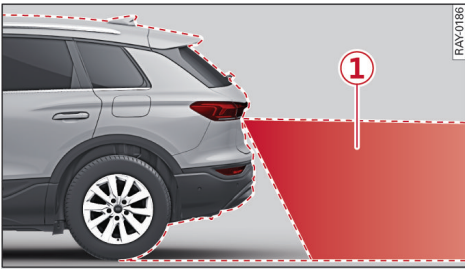
图 71 后视摄像头的探测范围
