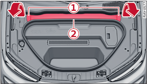
图 138 前舱：保险丝盒上方的盖子
