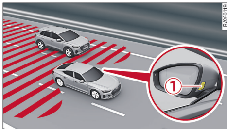
图 77 驾驶情形和外后视镜上的显示
