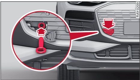
图 136 前保险杠：旋入拖车环
