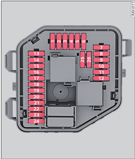
图 140 前舱右侧：保险丝座
