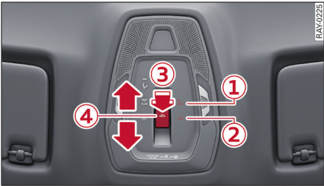
图 19 天花板：全景玻璃天窗和遮阳板按钮
