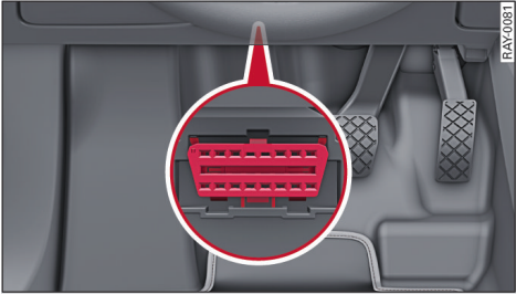
图 145 驾驶员侧的脚舱：诊断系统的接口
