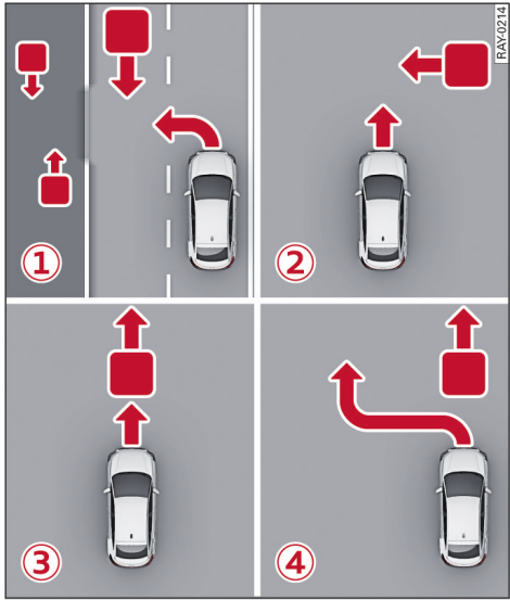
图 96 主动式前方辅助系统的功能（示例）
